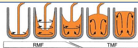
半凝固の模式図
